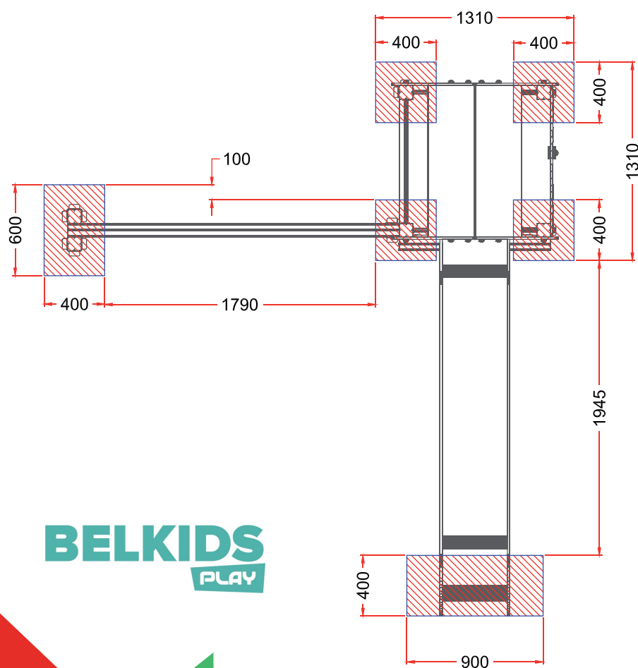
PLANTA CIMENTACION
