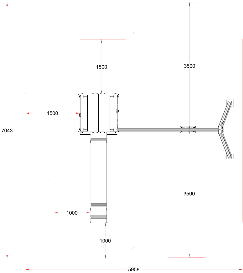
PLANTA
