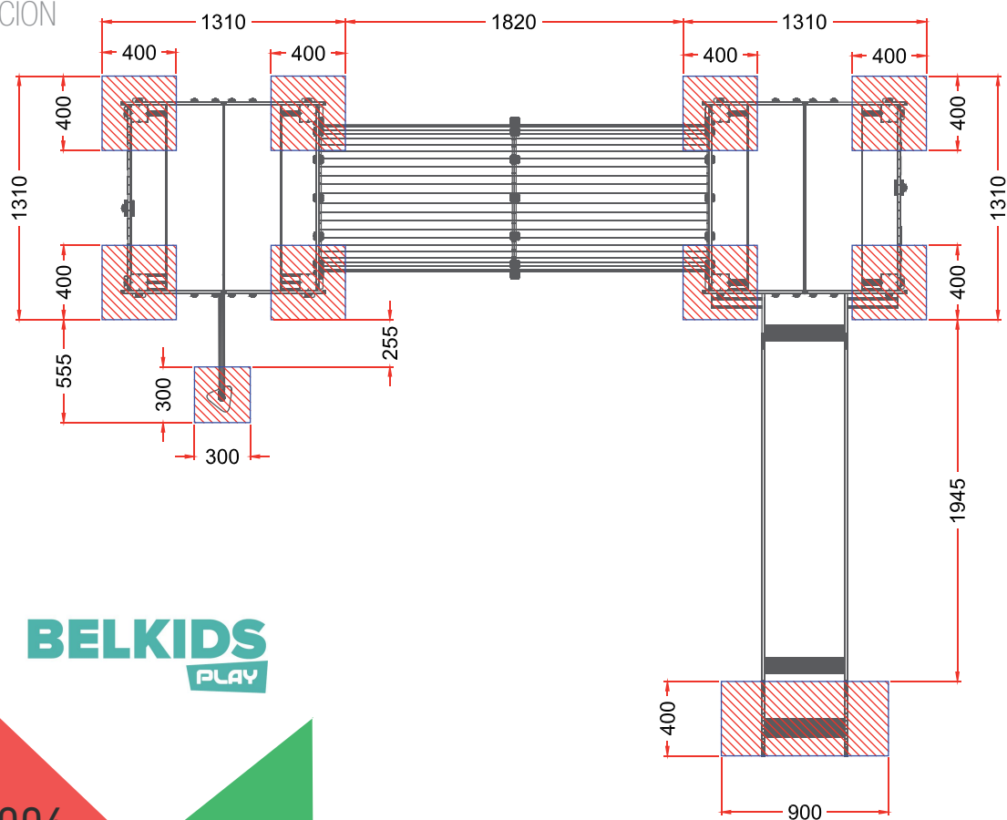
PLANTA CIMENTACION
