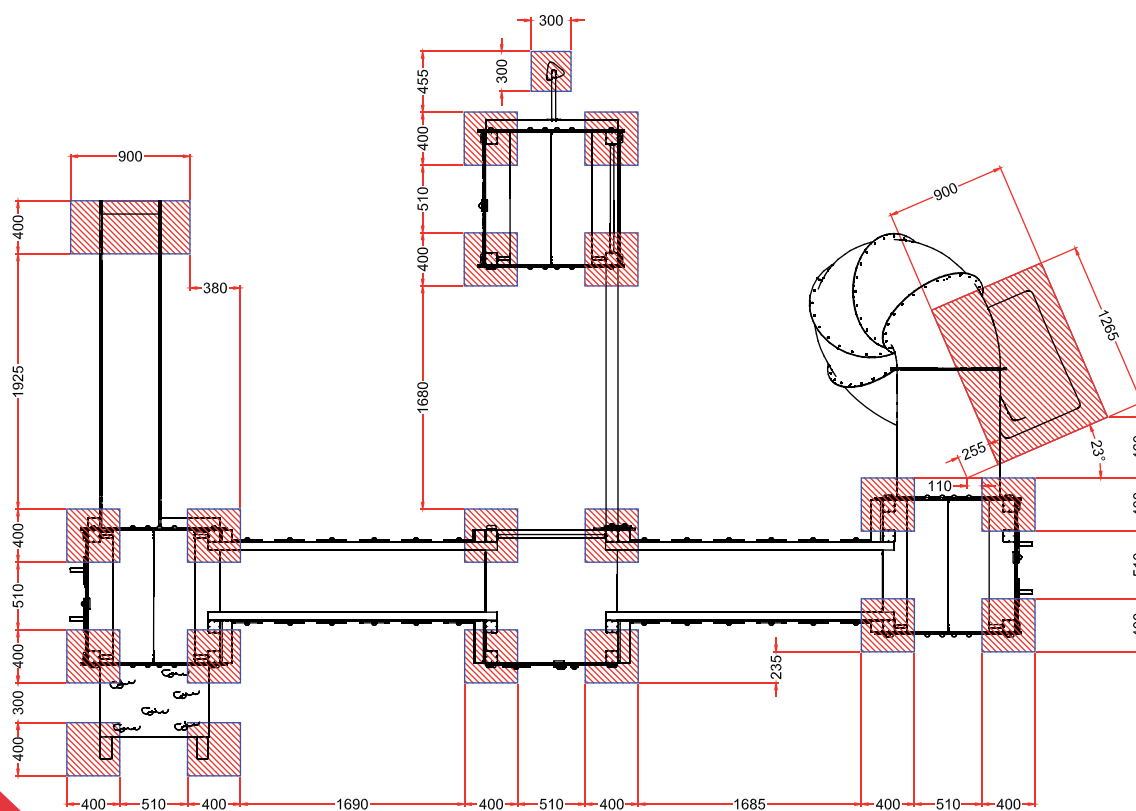
PLANTA CIMENTACION
