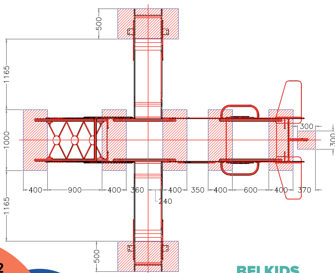
PLANTA CIMENTACION
