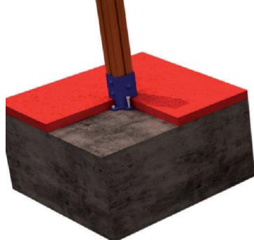
FIJACION A SOLERA DE HORMIGON
