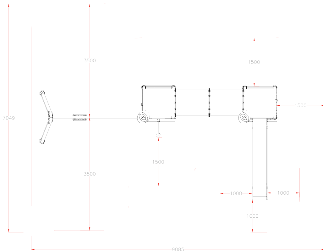
PLANTA
