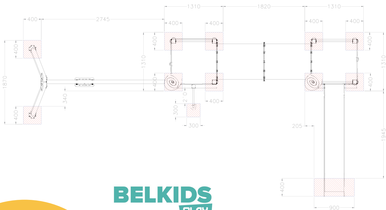
PLANTA CIMENTACION
