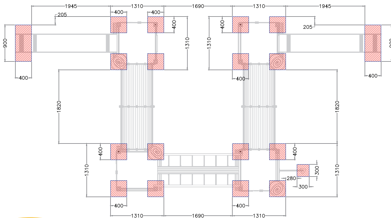
PLANTA CIMENTACION
