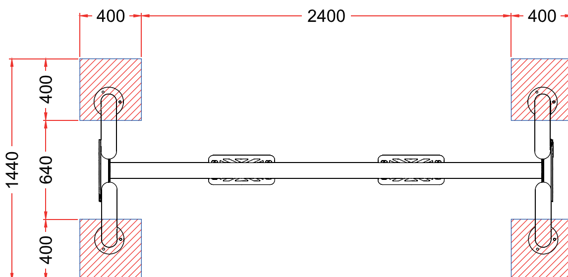
PLANTA CIMENTACION
