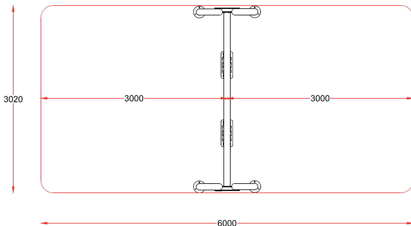
PLANTA
