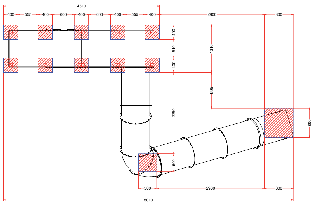
PLANTA CIMENTACION
