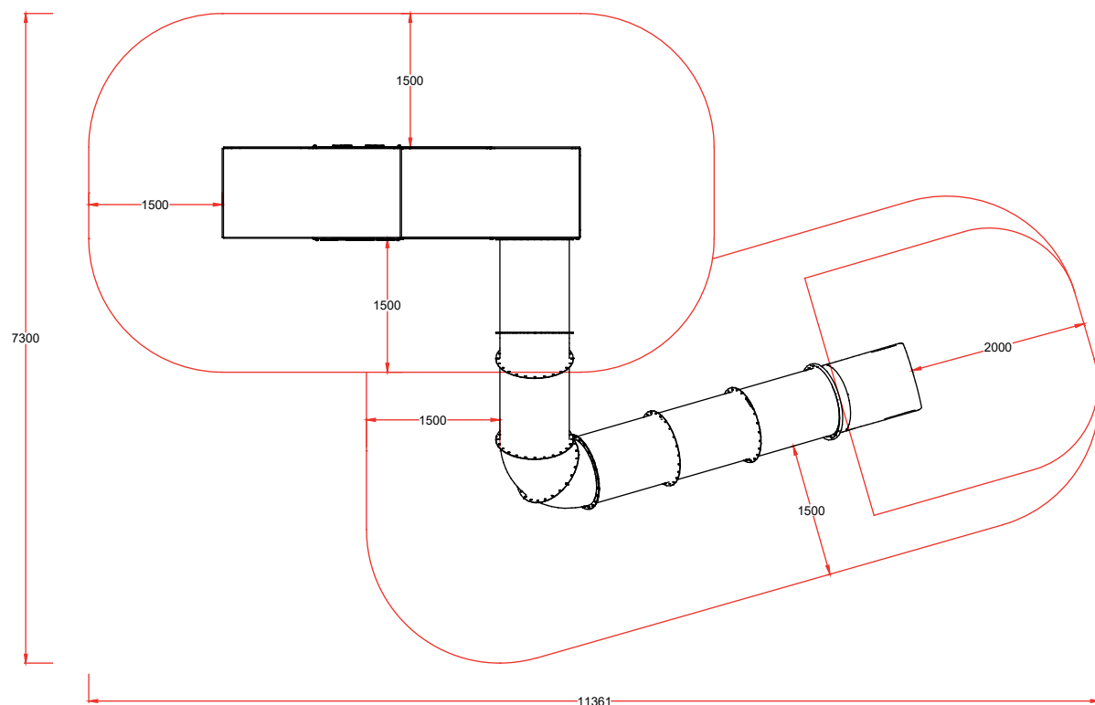
PLANTA
