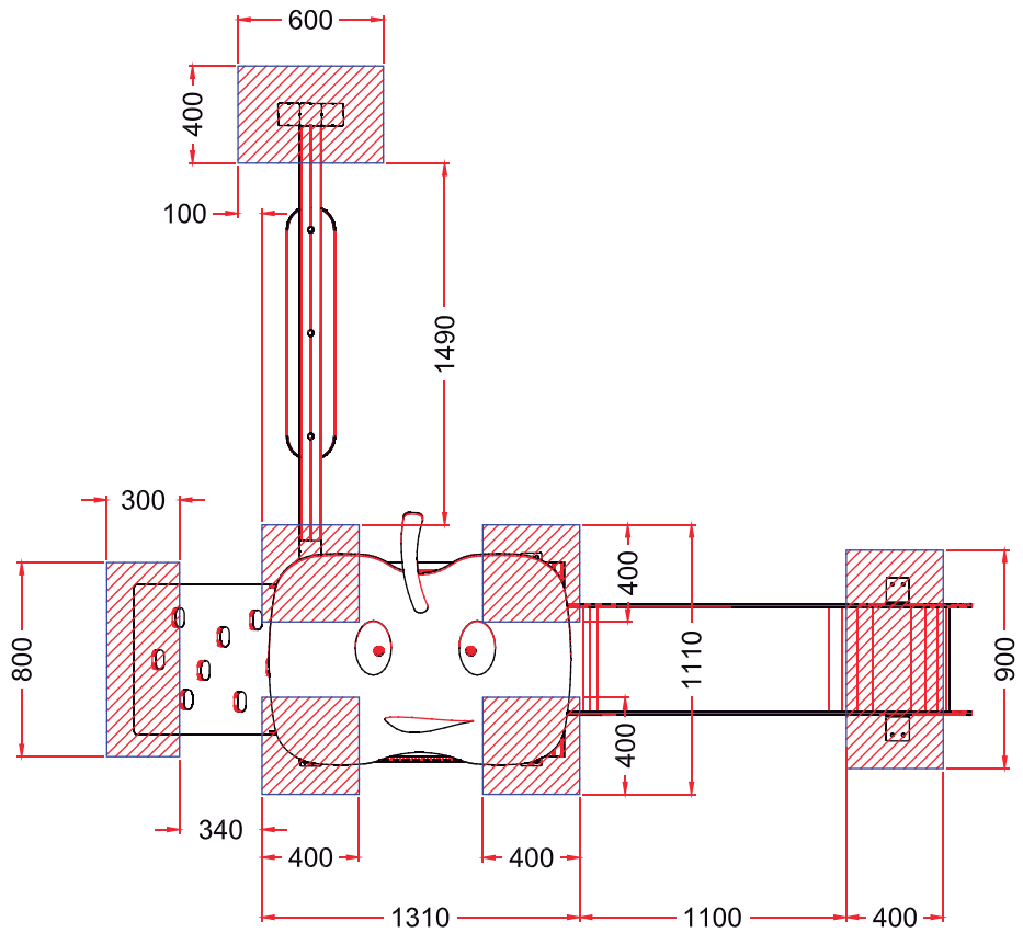
PLANTA CIMENTACION
