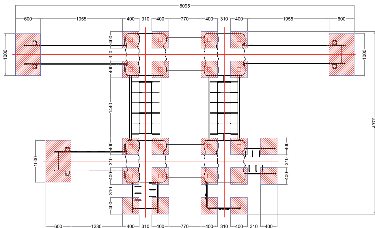
PLANTA CIMENTACION
