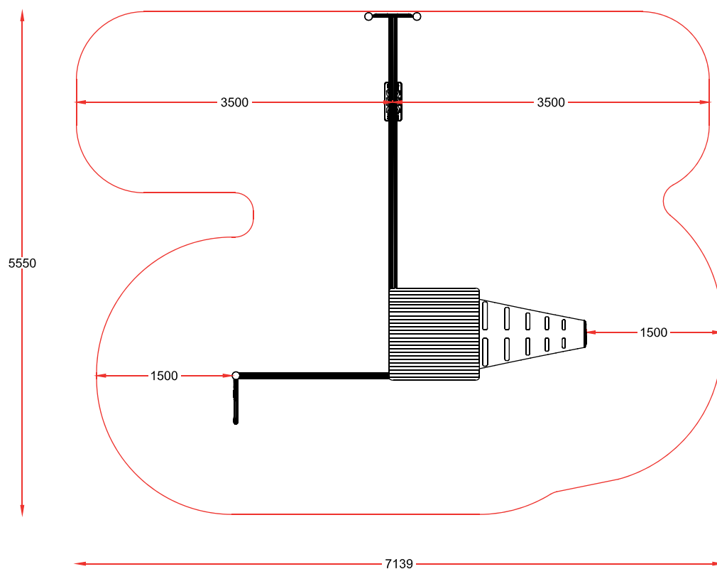
PLANTA CIMENTACION
