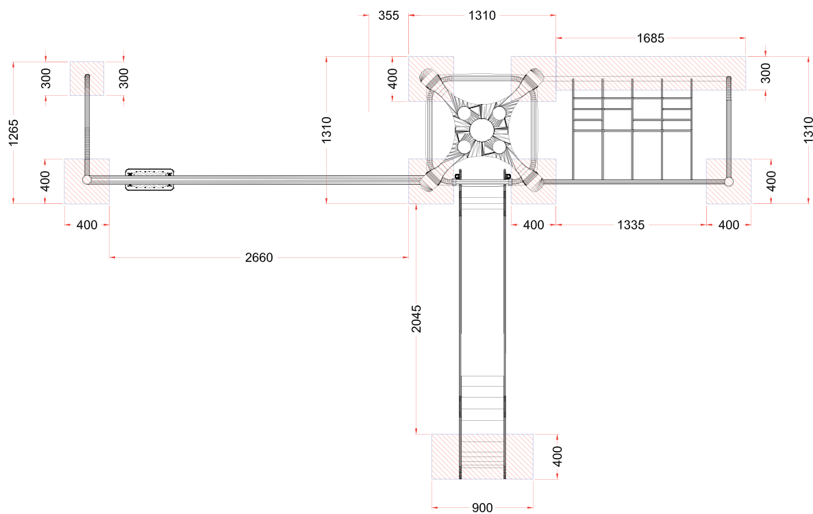
PLANTA CIMENTACION
