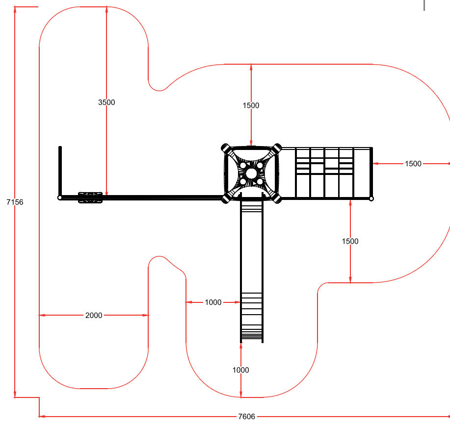
PLANTA
