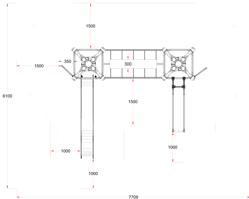
PLANTA CIMENTACION
