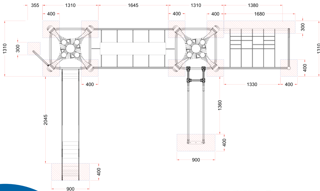
PLANTA CIMENTACION
