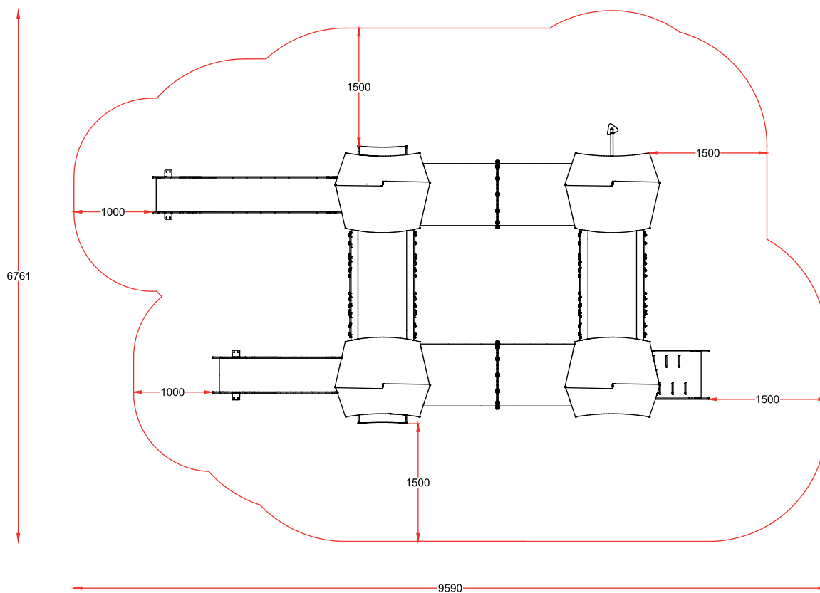
PLANTA CIMENTACION
