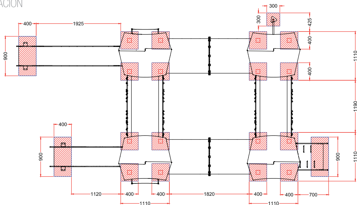
PLANTA CIMENTACION
