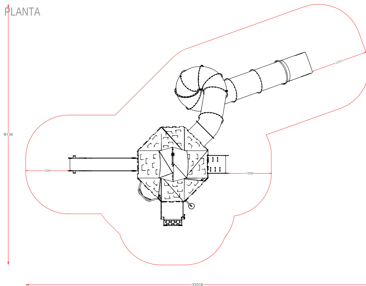
PLANTA CIMENTACION
