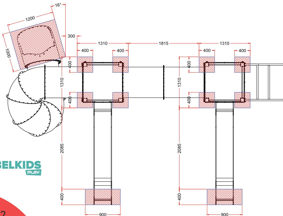
PLANTA CIMENTACION
